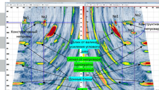
Контроль сварных швов мостовых конструкций
