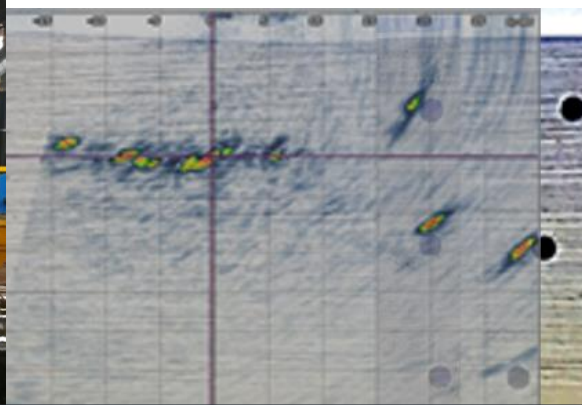
Контроль сварных швов эксцентриксов (УРБО)
