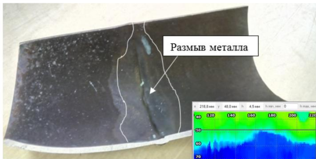
Фрагмент трубопровода АЭС
