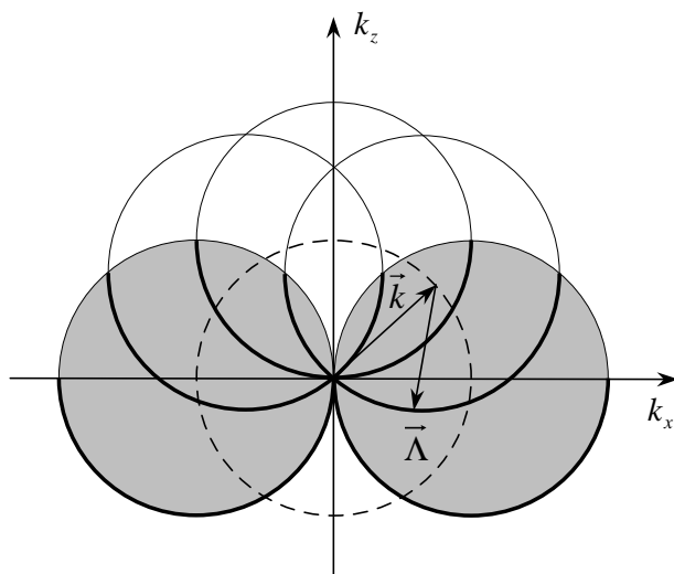
Рисунок 2 Структура данных в спектральном пространстве при работе «на просвет» в режиме двойного сканирования.
