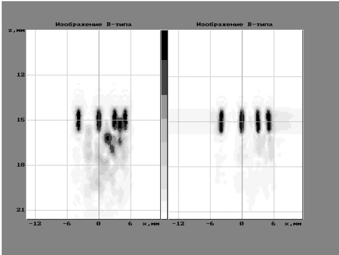
Рисунок 4 Изображение четыре точечных рассеивателей полученных методом ПСП и методом двойного сканирования. При расчете эхосигналов учитывалось четырехкратное перерассеивание и трансформация волн на точечных рассеивателях.
