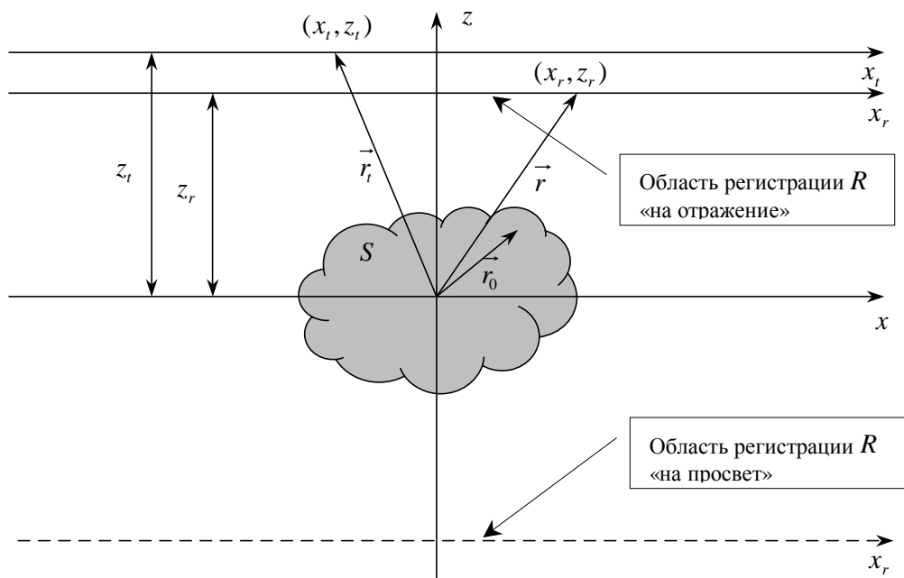
Рисунок 1 Схема проведения опыта в режиме двойного сканирования по измерению рассеянного поля излучателем и приемником, движущимся по линии независимо друг от друга.
