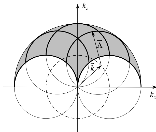
Рисунок 3 Структура данных в спектральном пространстве при работе «на отражение» в режиме двойного сканирования.
